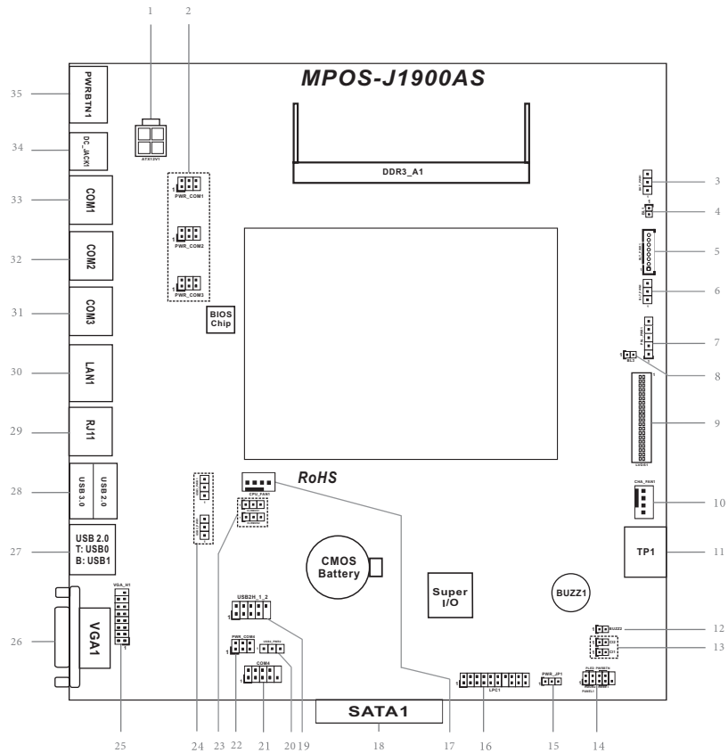
23 : Clear CMOS Headers
