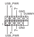
19 : USB2.0 Header (USB2H_1_2)
