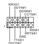
21 : COM Port Header (COM4) (RS232)
